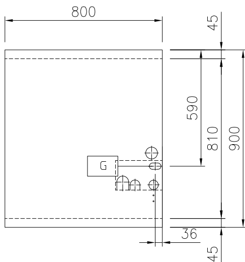
Boven aanzicht
